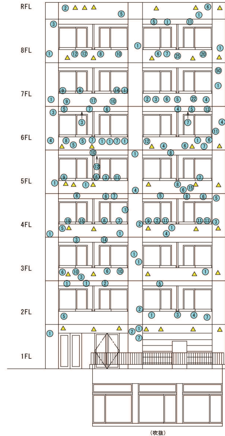
南立面図
