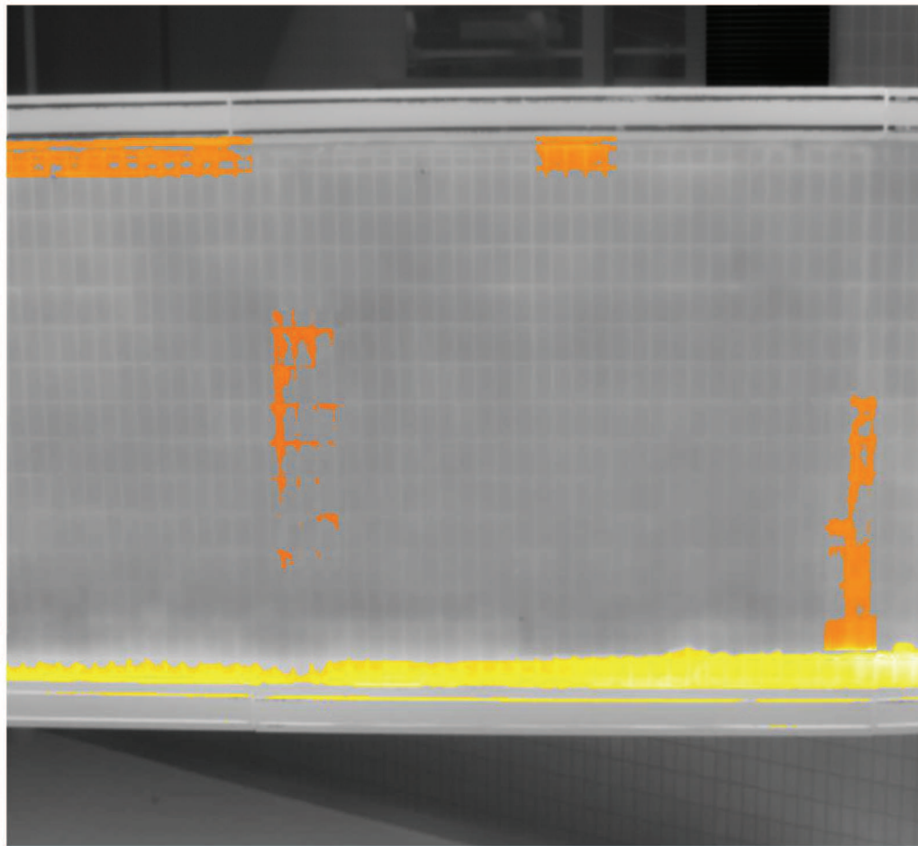
タイル浮きの兆候を示す温度分布有 003-0200
