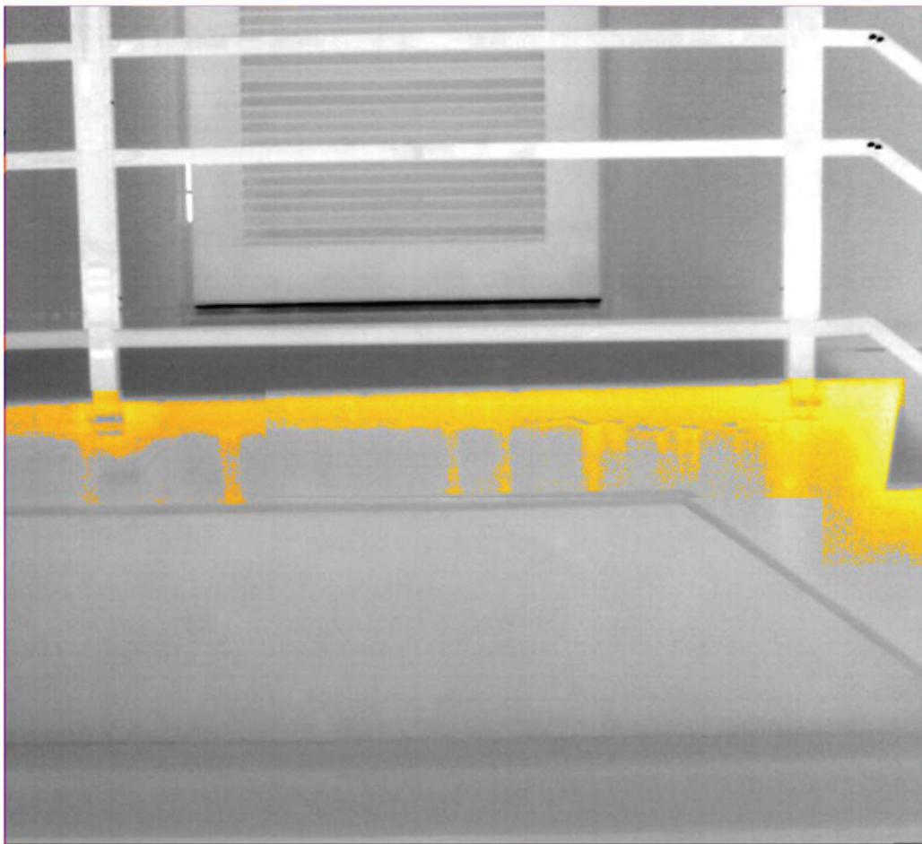
タイル浮きの兆候を示す温度分布有 004-0031
